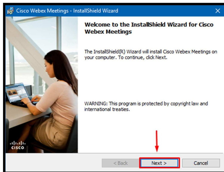
SLIKA 5 - PROCES INSTALCIJE
