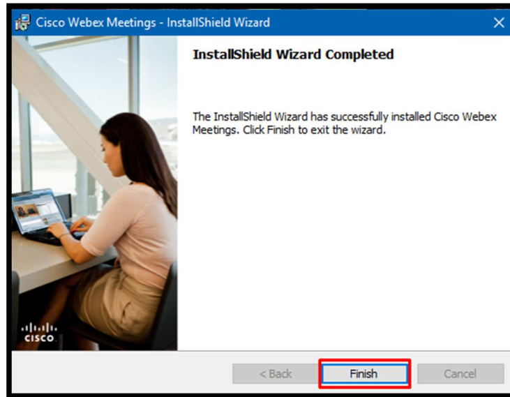
SLIKA 8 - ZAVRŠETAK INSTALACIJE
