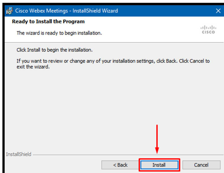
SLIKA 7 - POČETAK INSTALACIJE
