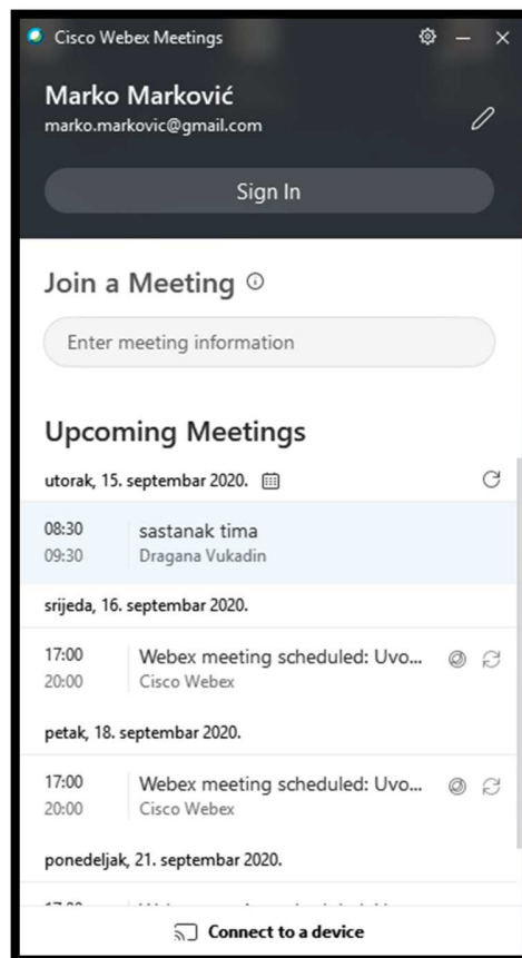
SLIKA 11 - POKRENUTA APLIKACIJA
